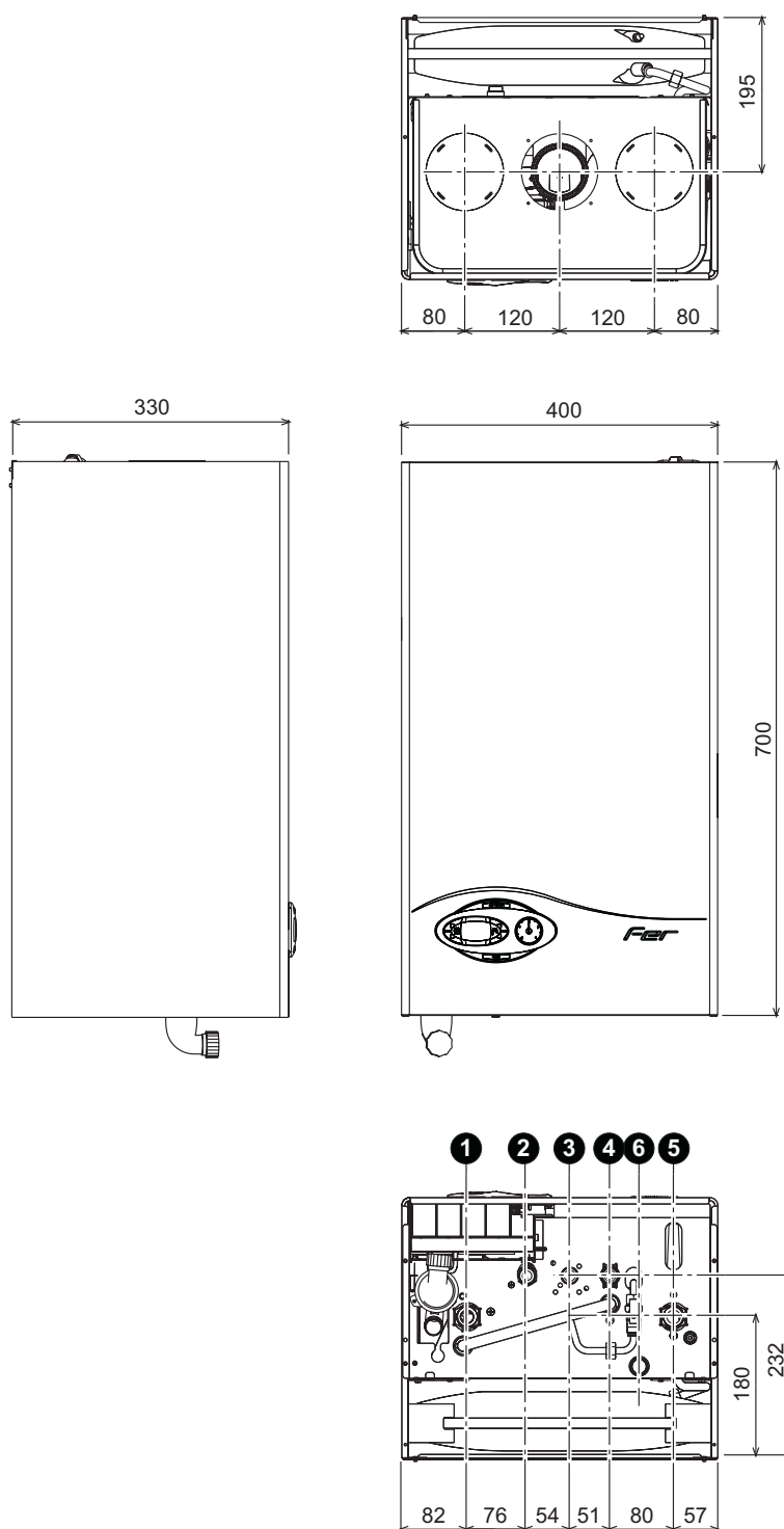
fig. 30 - Dimensioni e attacchi
