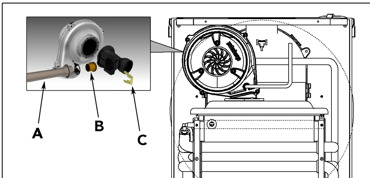
fig. 26 - Trasformazione gas
