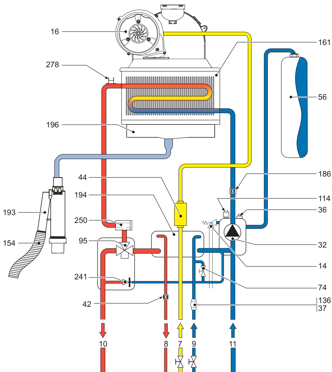
fig. 32 - Circuito idraulico
