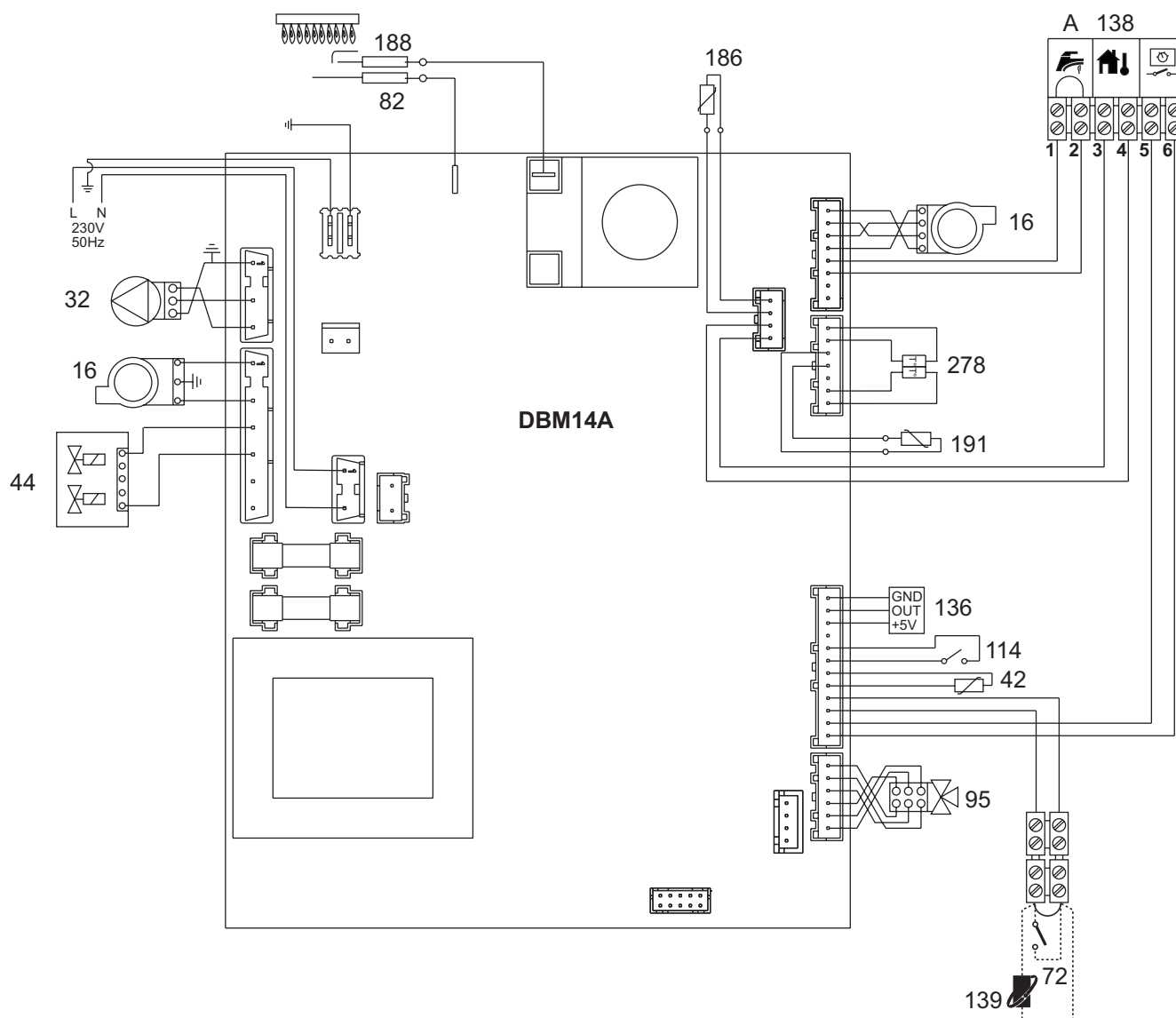
fig. 33 - Schema elettrico
